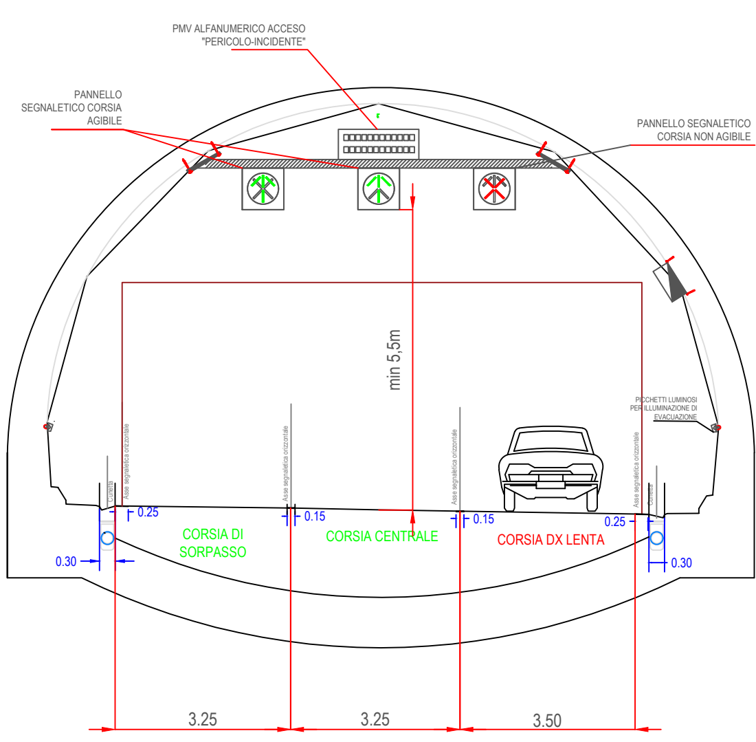
SEZIONE GALLERIA A-A' CASO INCIDENTE ORDINARIO scala 1:100
